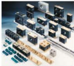
Befestigungsschelle DIN 3015 Collare fissaggio DIN 3015 Abrazadera DIN 3015
